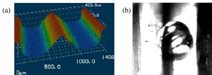
Figura 1. (a) superfície microestruturada vista em microscópio confocal e (b) bolha nucleando em um microcanal.
